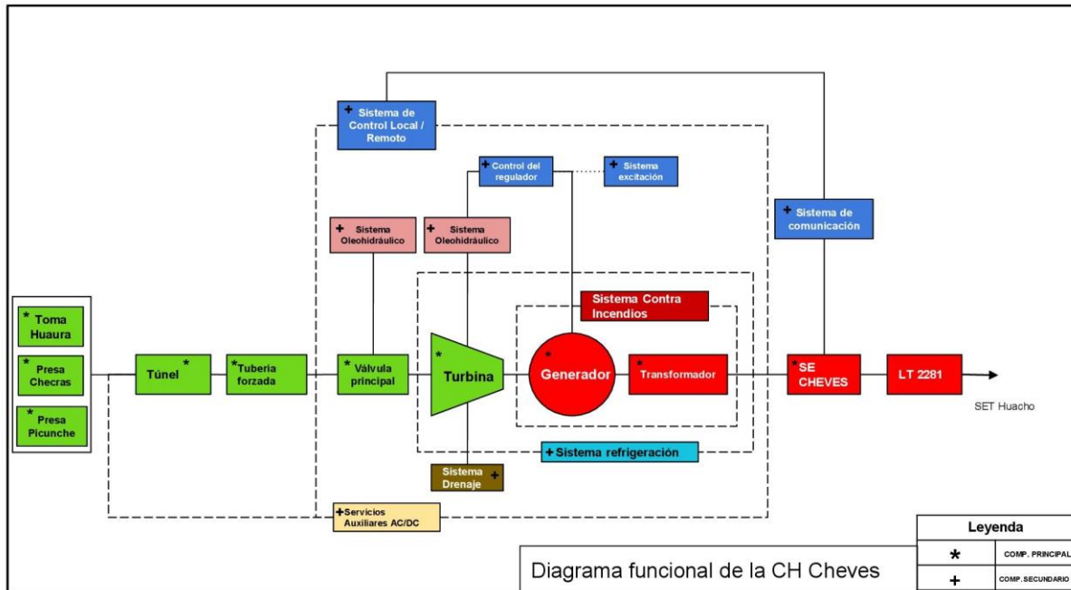
Figura Nº 1. Diagrama de flujo de la CH Cheves
