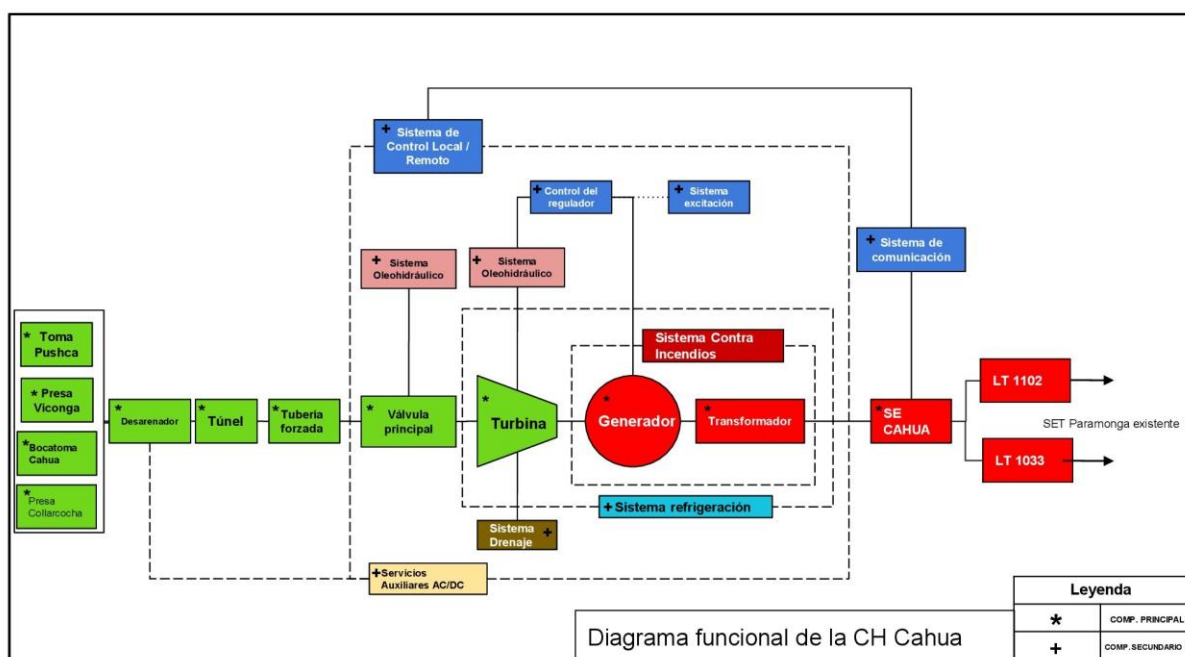
Figura N° 1. Diagrama de flujo de la CH Cahua
