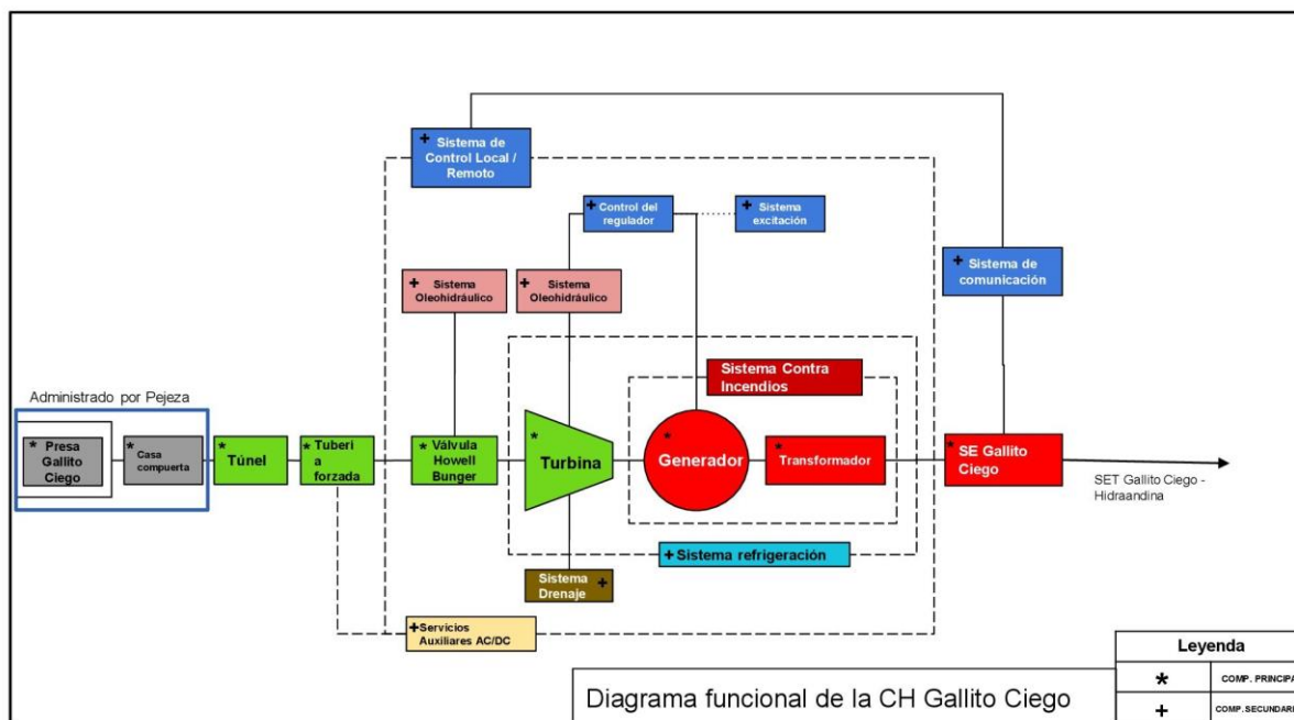
Figura N° 1. Diagrama de flujo de la CH Gallito Ciego
